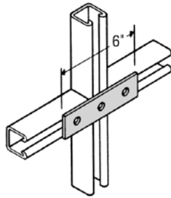
CS-101 3 Hole Flat
