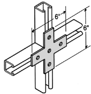
CS-111 Flat Cross
