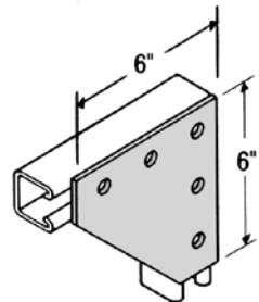
CS-115 5 Hole Heavy Duty L
